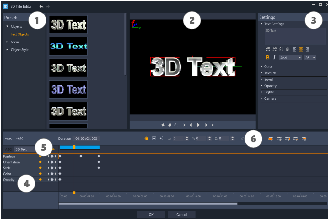
Области Редактора 3D титров: 1. Панель шаблонов; 2. Панель проигрывателя; 3. Панель настроек; 4. Панель шкалы времени; 5. Список объектов (Слои); 6. Панель инструментов временной шкалы
